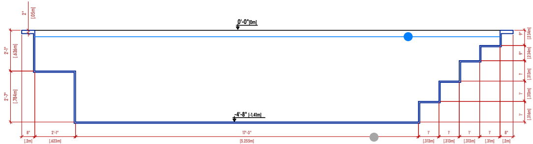
CORTE LONGITUDINAL | LONGITUDINAL SECTION | SECTION LONGITUDINALE
