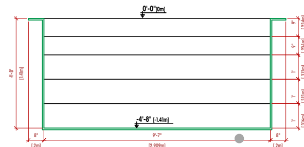
CORTE TRANSVERSAL | CROSS SECTION | LA COUPE TRANSVERSALE
