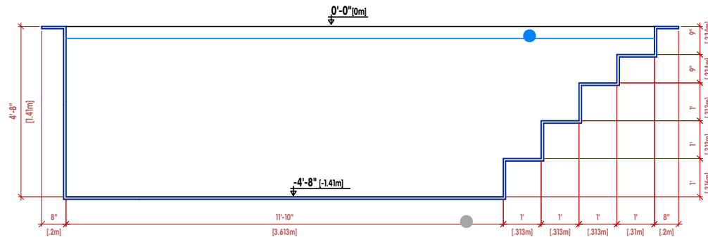
CORTE LONGITUDINAL | LONGITUDINAL SECTION | SECTION LONGITUDINALE
