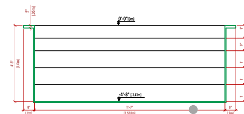
CORTE TRANSVERSAL
