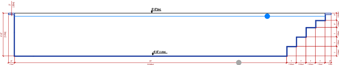
CORTE LONGITUDINAL | LONGITUDINAL SECTION | SECTION LONGITUDINALE
