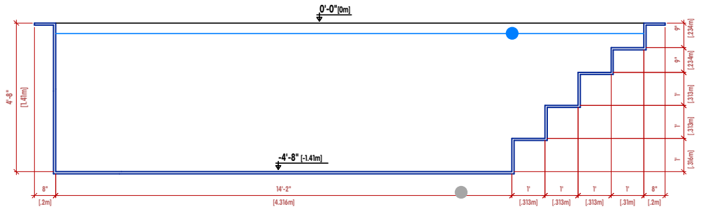
CORTE LONGITUDINAL | LONGITUDINAL SECTION | SECTION LONGITUDINALE
