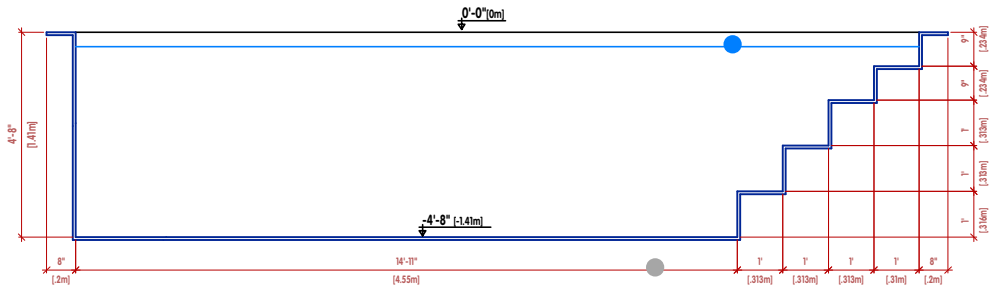
CORTE LONGITUDINAL |LONGITUDINAL SECTION|SECTION LONGITUDINALE
