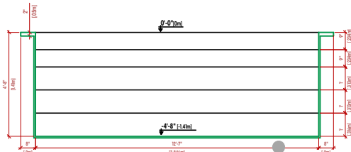
CORTE TRANSVERSAL | CROSS SECTION | LA COUPE TRANSVERSALE
