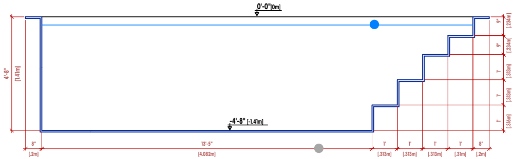
CORTE LONGITUDINAL | LONGITUDINAL SECTION | SECTION LONGITUDINALE
