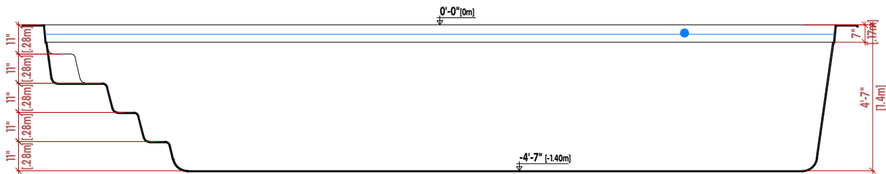
● CORTE LONGITUDINAL | LONGITUDINAL SECTION | SECTION LONGITUDINALE
