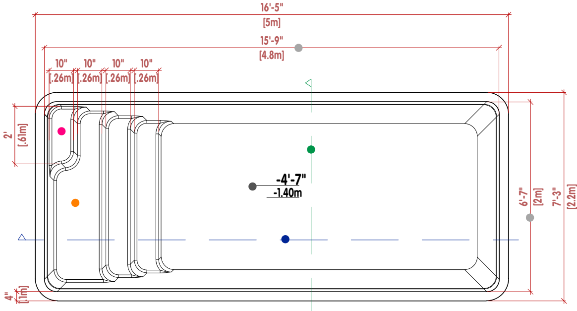
DESENHO TÉCNICO |TECHNICAL DESIGN|DIBUJO TÉCNICO|DESSINS TECHNIQUES
