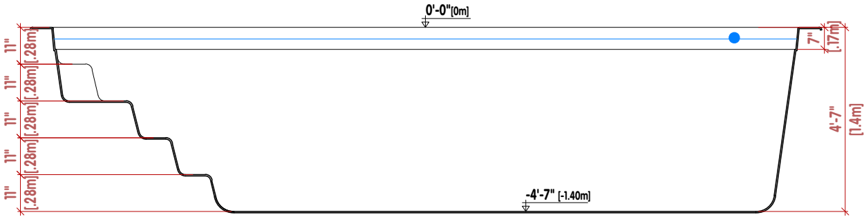
● CORTE LONGITUDINAL |LONGITUDINAL SECTION| SECTION LONGITUDINALE
