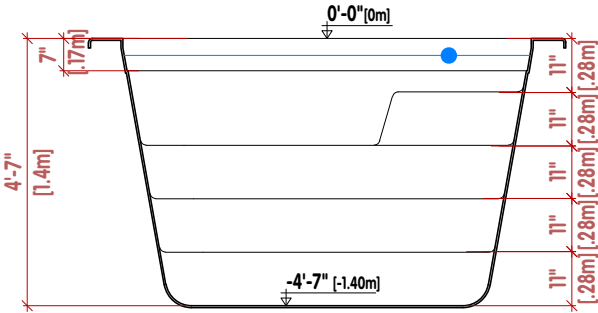
● CORTE TRANSVERSAL |CROSS SECTION| LA COUPE TRANSVERSALE
