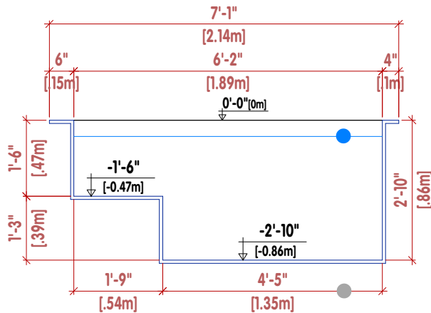
CORTE LONGITUDINAL | LONGITUDINAL SECTION | SECTION LONGITUDINALE
