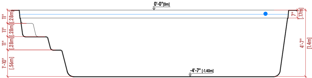
CORTE LONGITUDINAL | LONGITUDINAL SECTION | SECTION LONGITUDINALE
