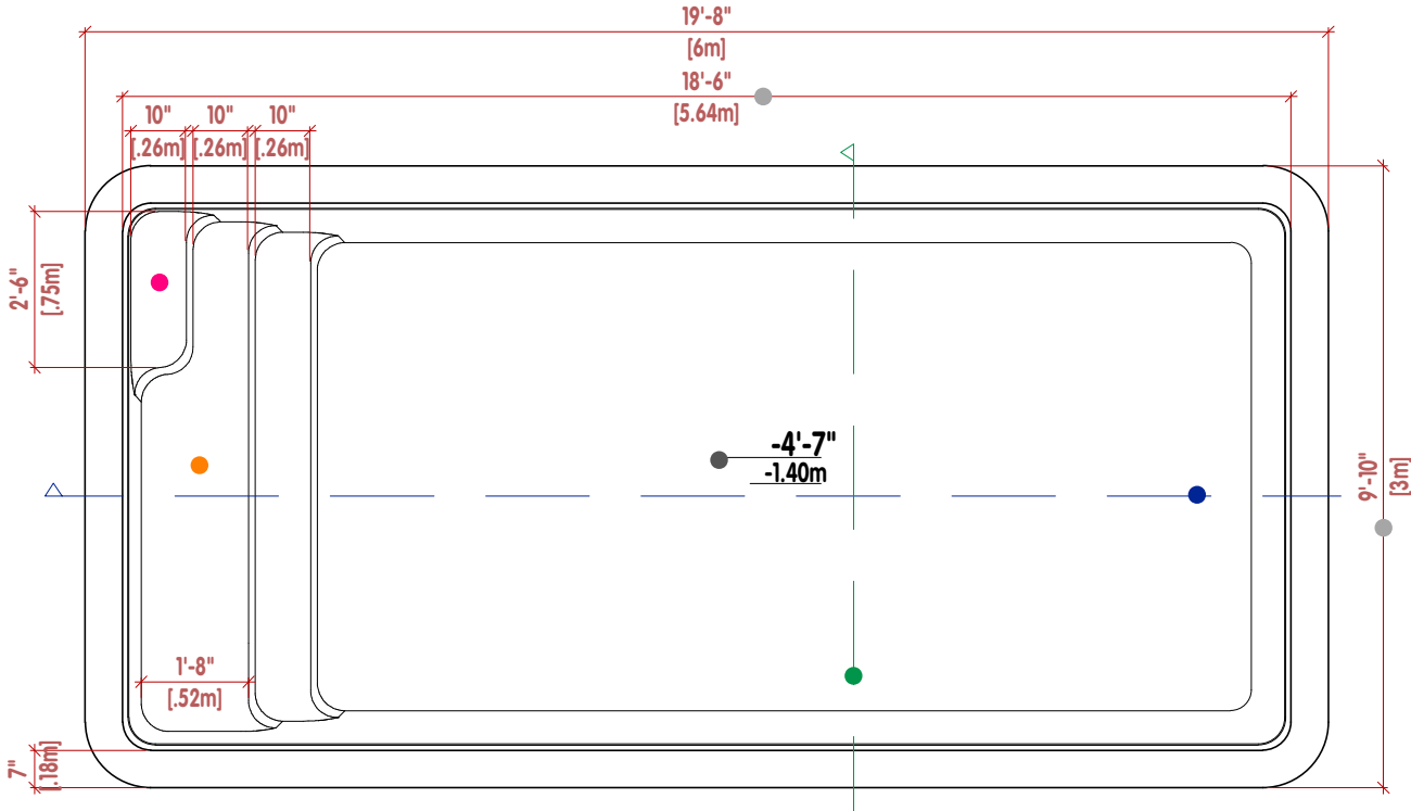
DESENHO TÉCNICO
