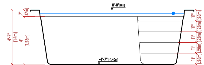
● CORTE TRANSVERSAL |CROSS SECTION| LA COUPE TRANSVERSALE
