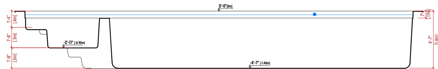
● CORTE LONGITUDINAL | LONGITUDINAL SECTION | SECTION LONGITUDINALE
