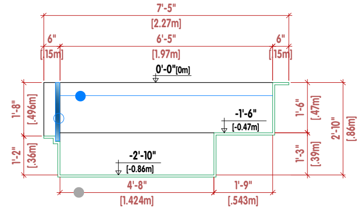
CORTE TRANSVERSAL | CROSS SECTION | LA COUPE TRANSVERSALE
