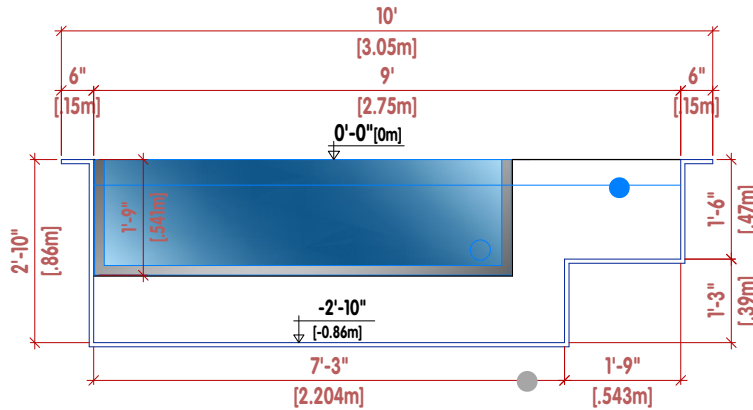
CORTE LONGITUDINAL | LONGITUDINAL SECTION | SECTION LONGITUDINALE
