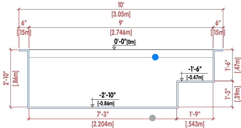
CORTE LONGITUDINAL | LONGITUDINAL SECTION | SECTION LONGITUDINALE
