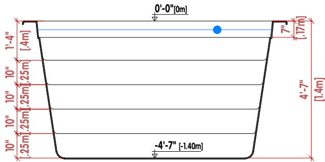
CORTE TRANSVERSAL
