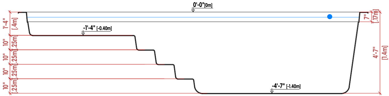
CORTE LONGITUDINAL
