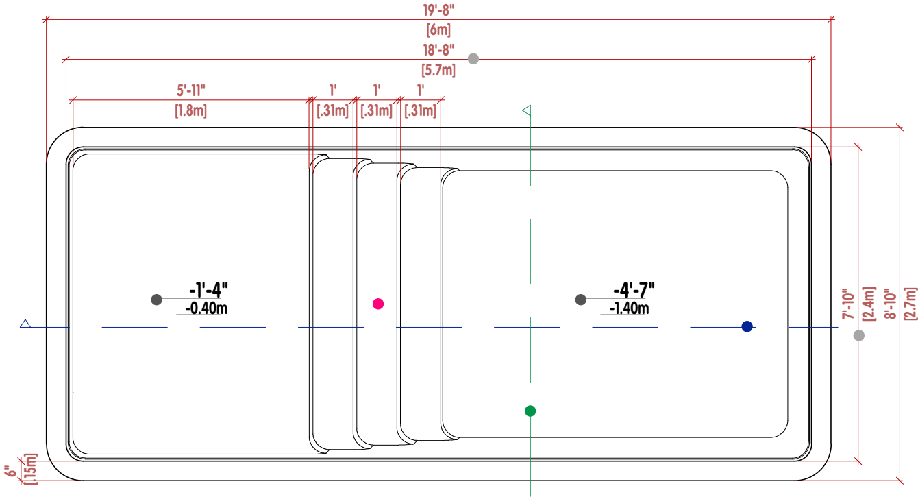
DESENHO TÉCNICO
