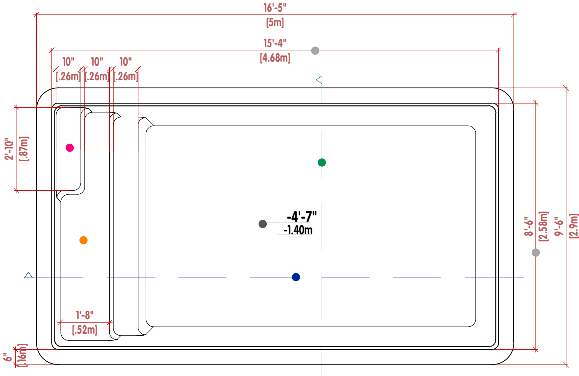
DESENHO TÉCNICO |TECHINICAL DESIGN|DIBUJO TÉCNICO|DESSINS TECHNIQUES
