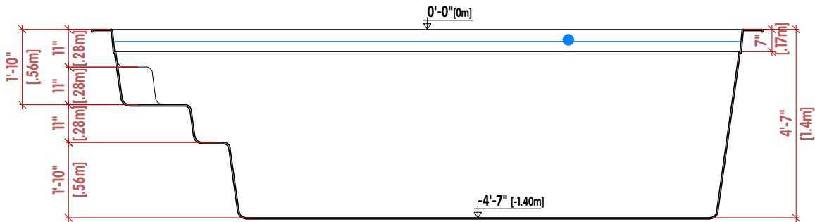
● CORTE LONGITUDINAL |LONGITUDINAL SECTION|SECTION LONGITUDINALE
