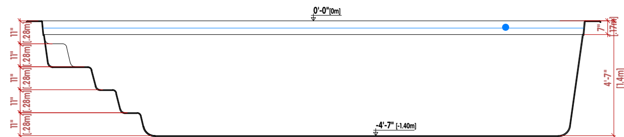
● CORTE LONGITUDINAL |LONGITUDINAL SECTION|SECTION LONGITUDINALE
