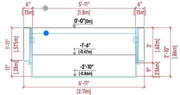
CORTE TRANSVERSAL | CROSS SECTION | LA COUPE TRANSVERSALE
