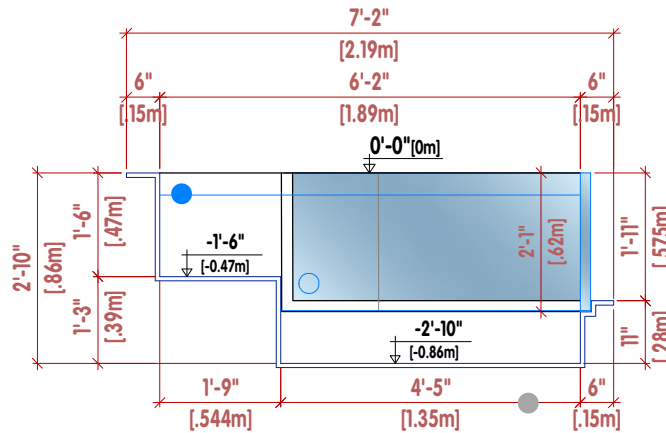
CORTE LONGITUDINAL | LONGITUDINAL SECTION | SECTION LONGITUDINALE
