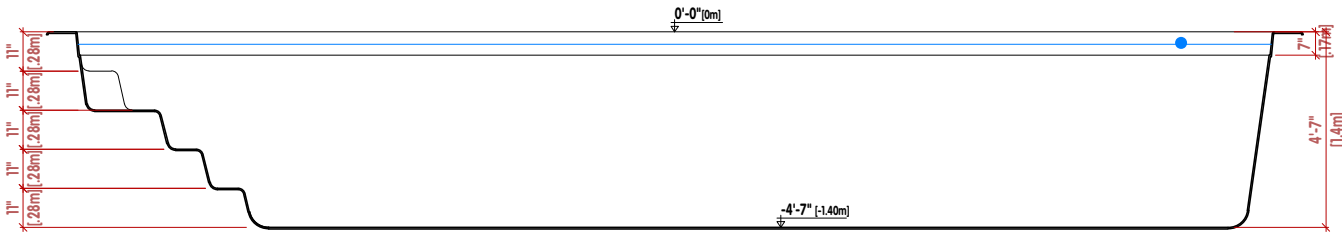
● CORTE LONGITUDINAL | LONGITUDINAL SECTION | SECTION LONGITUDINALE
