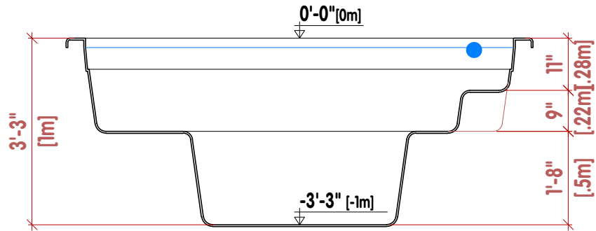
DESENHO TÉCNICO | TECHNICAL DESIGN | DIBUJO TÉCNICO | DESSINS TECHNIQUES
