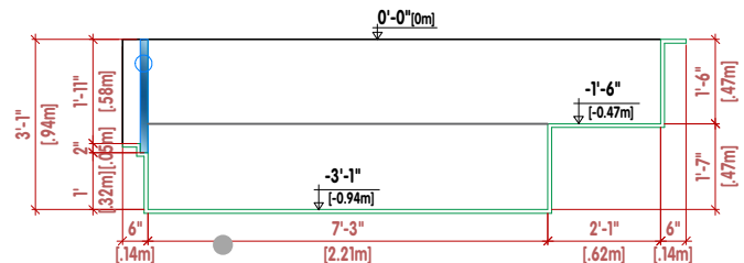
CORTE TRANSVERSAL | CROSS SECTION | LA COUPE TRANSVERSALE
