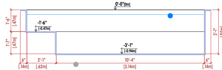
CORTE LONGITUDINAL | LONGITUDINAL SECTION | SECTION LONGITUDINALE
