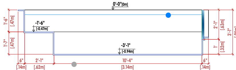
CORTE LONGITUDINAL | LONGITUDINAL SECTION | SECTION LONGITUDINALE
