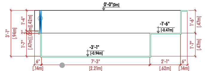
CORTE TRANSVERSAL |CROSS SECTION| LA COUPE TRANSVERSALE
